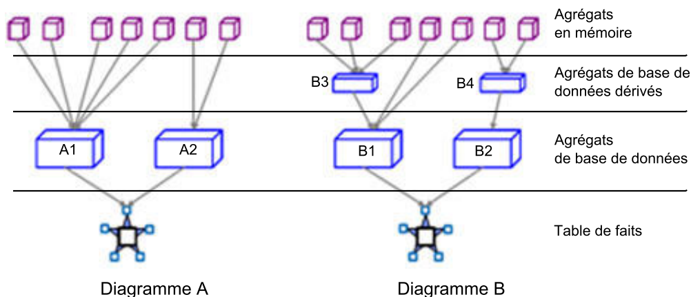
Figure 1. Recommandations d'agrégat dérivées d'une table de faits et d'autres agrégats de base de données
